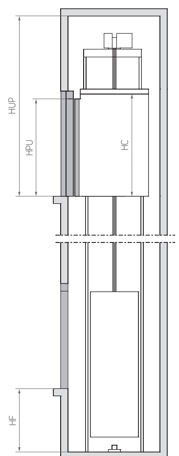
VERTICALE DOORSNEDE
